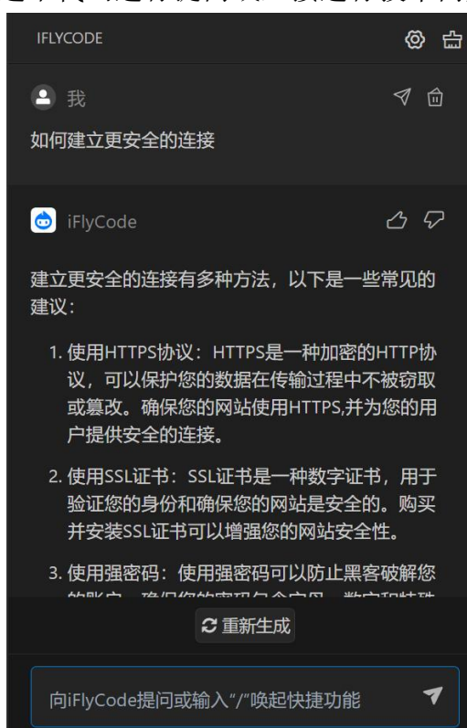
图 12 知识问答
