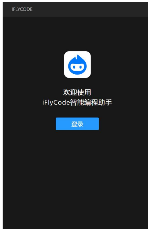
图 4 插件登录
